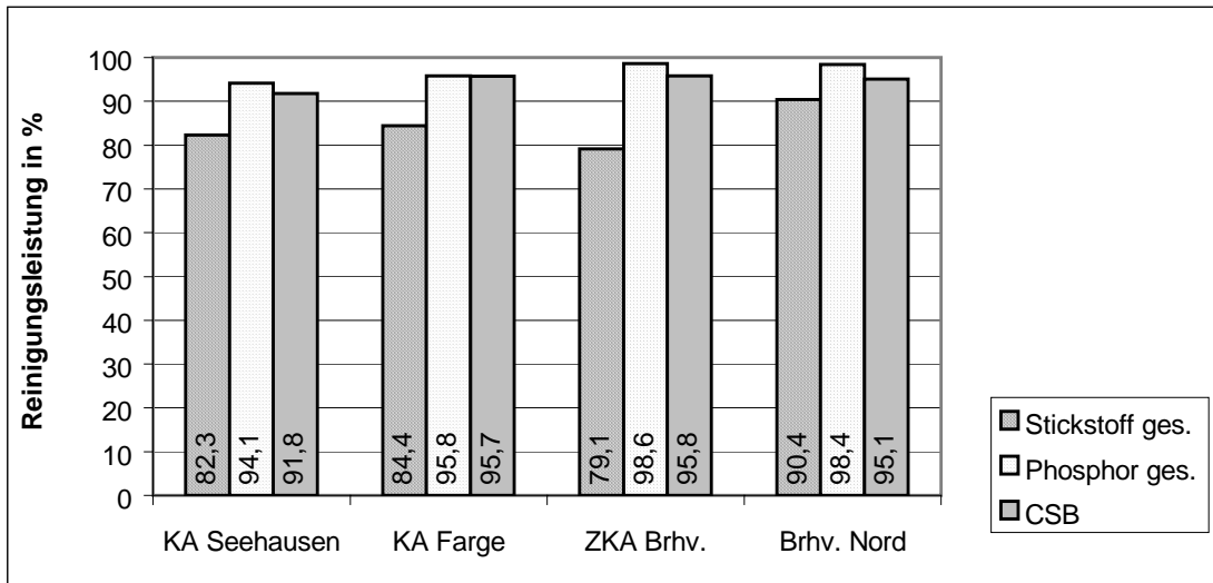
Abbildung 2: Reinigungsleistung der Kläranlagen
