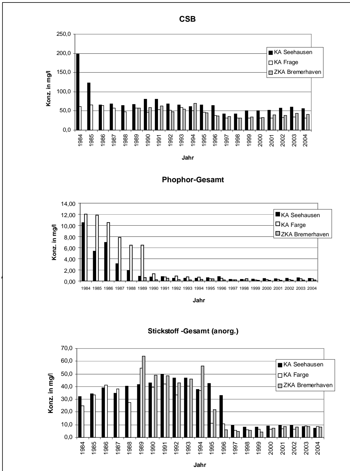
Abbildung 2: Ablaufkonzentrationen kommunaler Großkläranlagen (Werte ZKA Bhv liegen erst ab erst 1989 vor)
