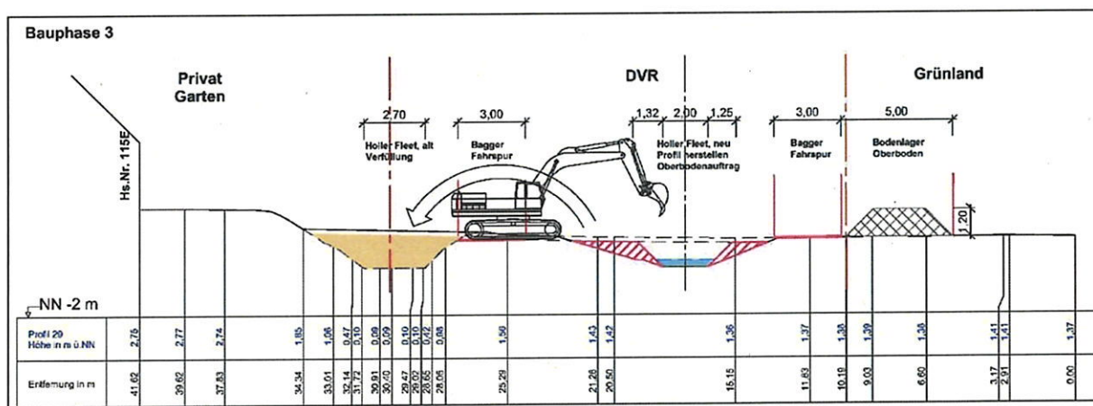
Abbildung 23: Schnitt Prinzip Baudurchführung Bauphase 3 (Profil 29)
