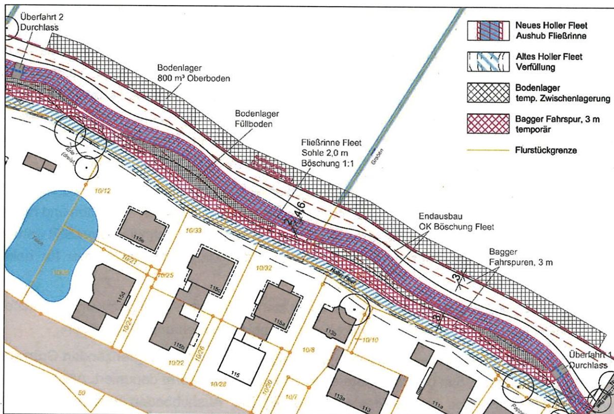
Abbildung 21: Lageplan Prinzip Baudurchführung Bauphase 1 (südöstlicher Abschnitt)
