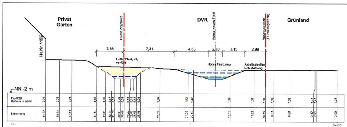
Abbildung 19: Gewässerprofil 29 – (l) altes und (r) neues Fleet
