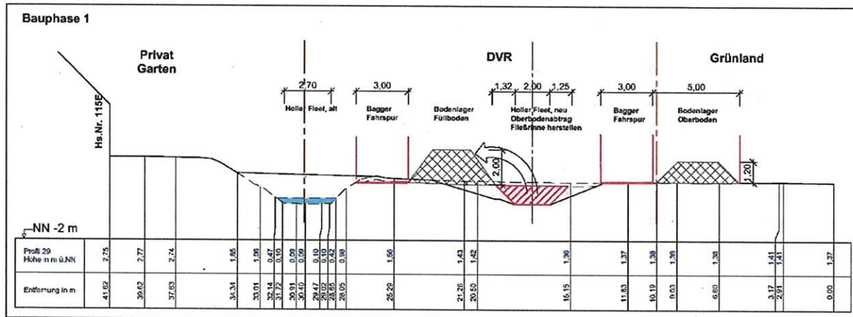
Abbildung 20: Schnitt Prinzip Baudurchführung Bauphase 1 (Profil 29)
