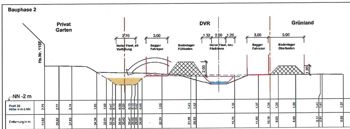
Abbildung 22: Schnitt Prinzip Baudurchführung Bauphase 2 (Profil 29)
