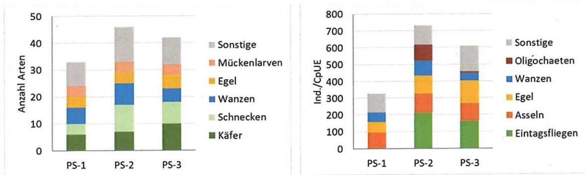
Abbildung 17: Artenzahlen (links) und Abundanzen (rechts) des Makrozoobenthos an den Probestellen im Holler Fleet.
