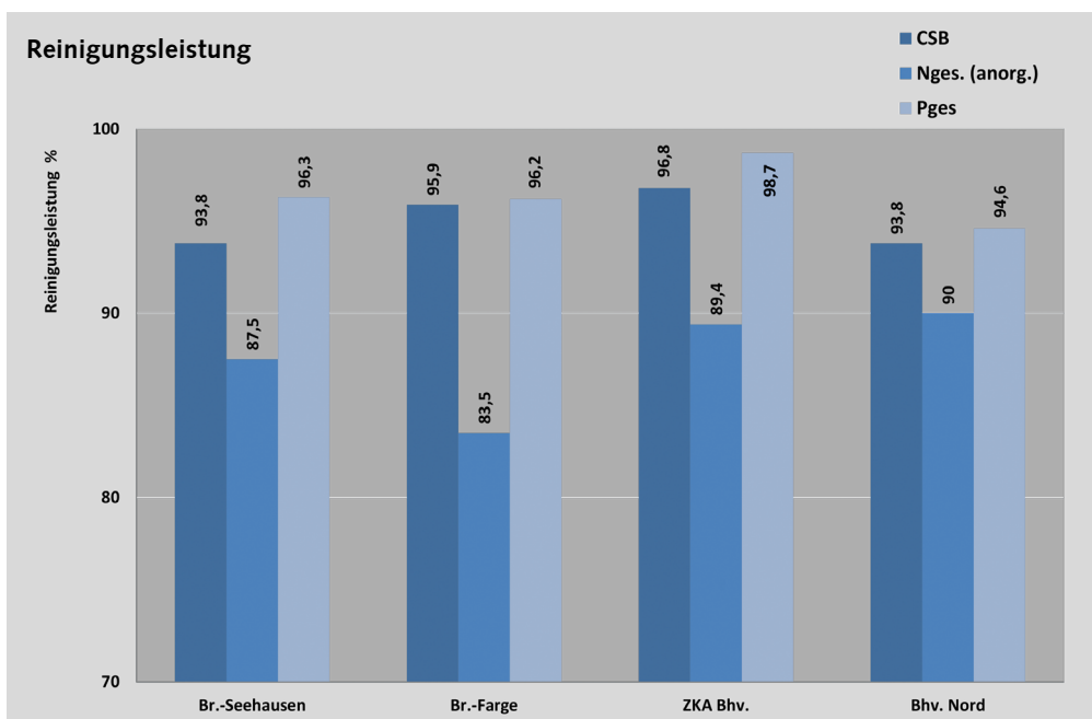
Abbildung 3: Reinigungsleistung [%] der Kläranlagen
