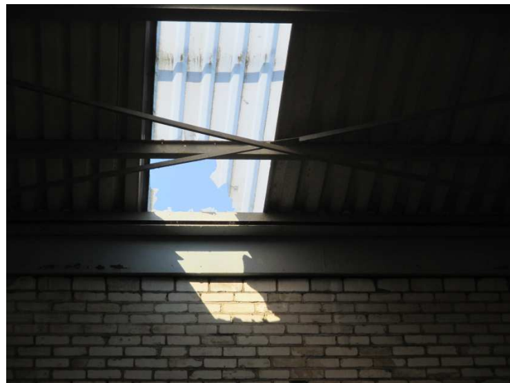
Abb. 2: Durchsturzstelle, Höhe ca. 7m
