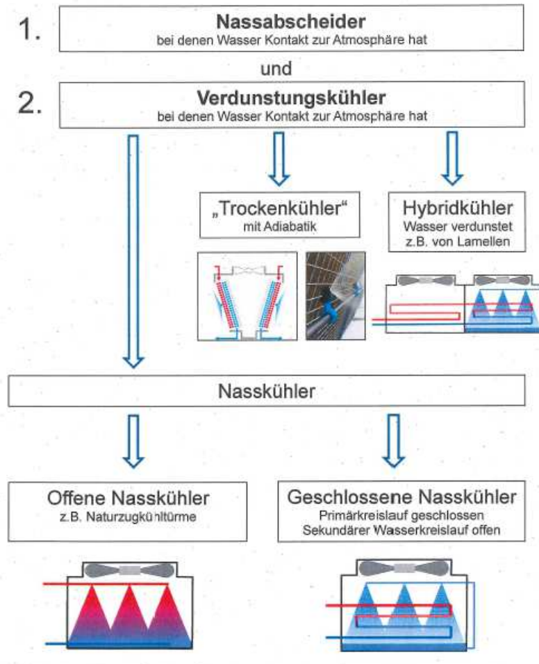
Abb. 3: Verschiedene Typen von Verdunstungskühlern. Gegenstand der 42. BImSchV und der VDI 2047
