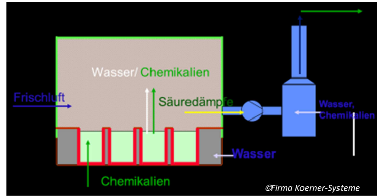
Abb. 1: Prinzipskizze des Gaswäschers
