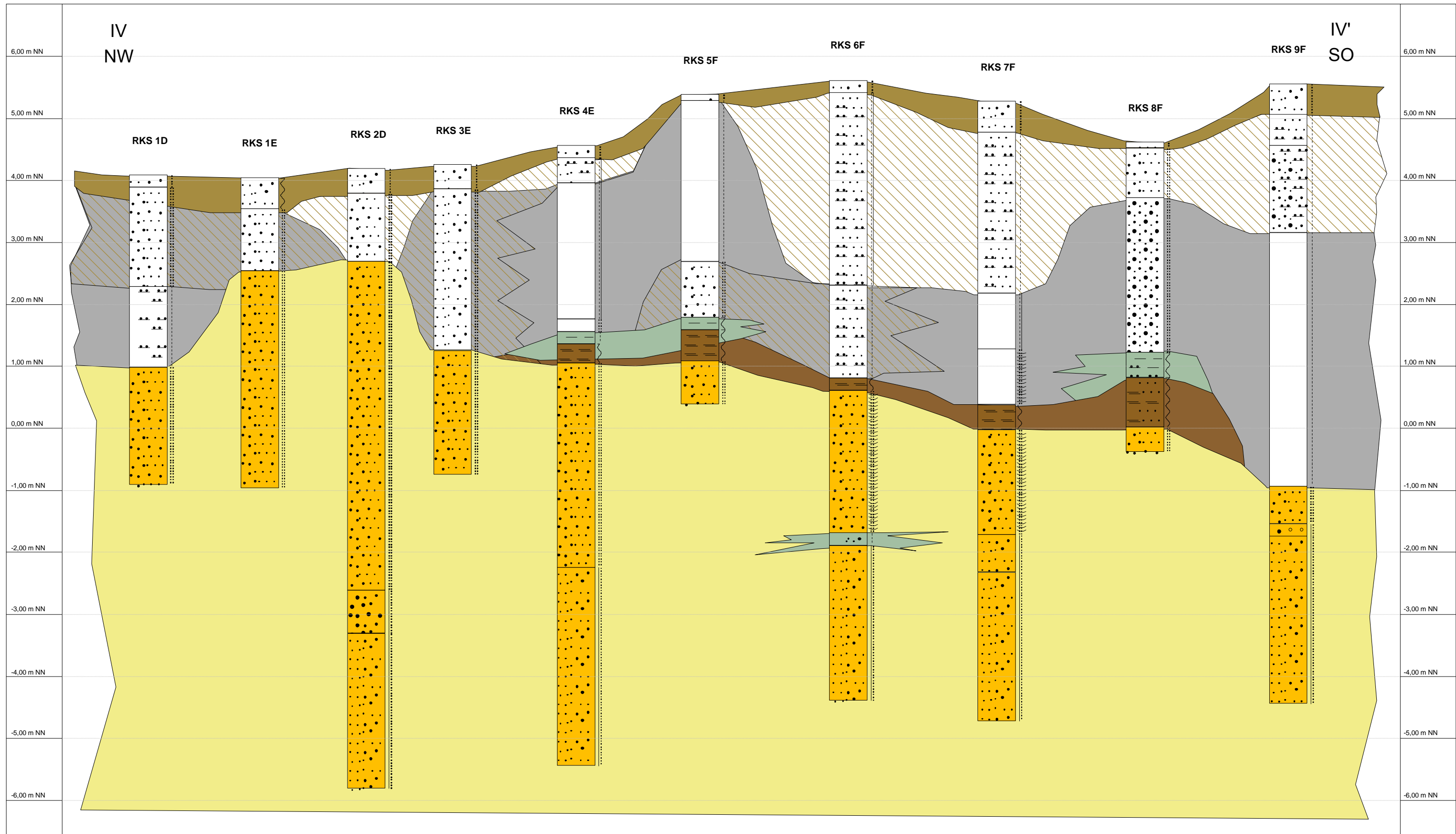
Anlage 4.5 Profilschnitt IV - IV'
