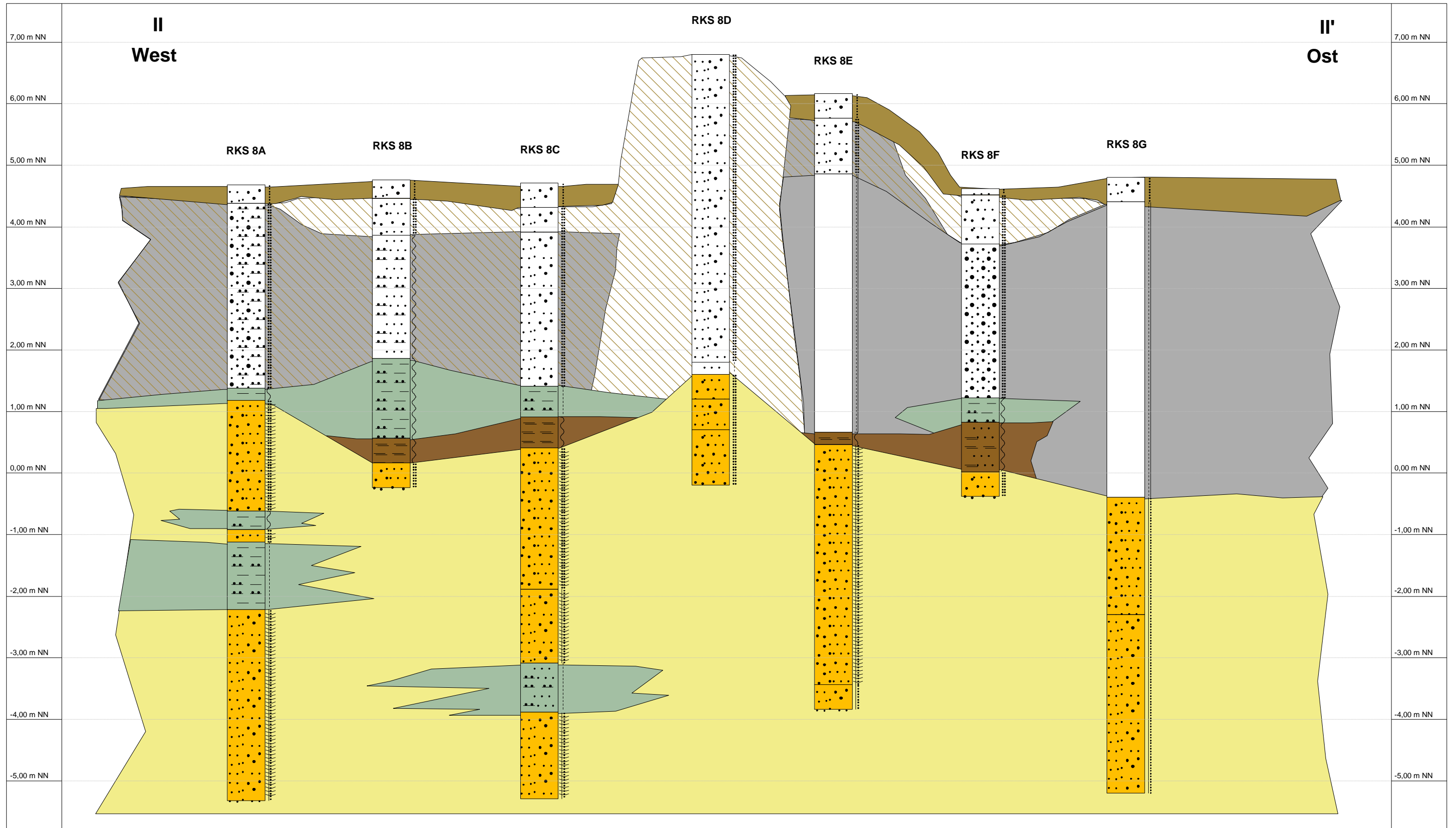
Anlage 4.3 Profilschnitt II - II'
