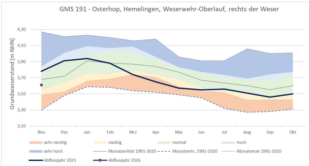
Abbildung 12- Monatliche Mittelwerte Grundwasserstand, Grundwassermessstelle Osterhop, Hemelingen
