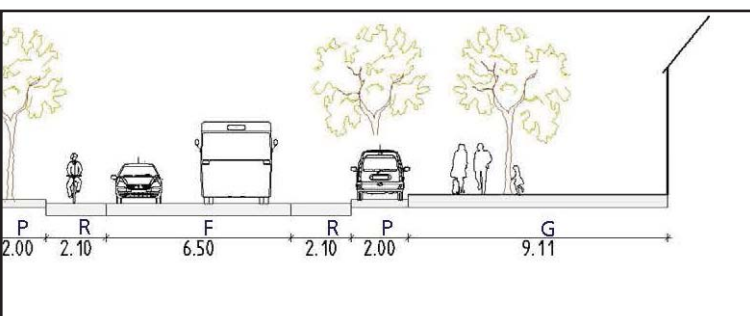
Straßenquerschnitt Steffensweg
